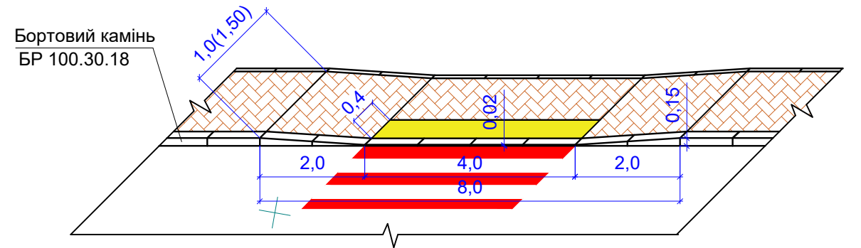
Схема пониження бортового каменю на пішохідних переходах
